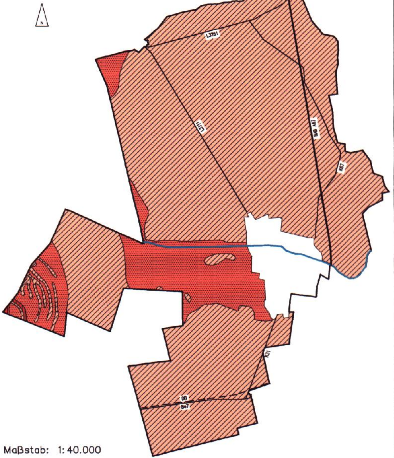
Abb. 4: Grundwasserschutzfunktion Nitrat
