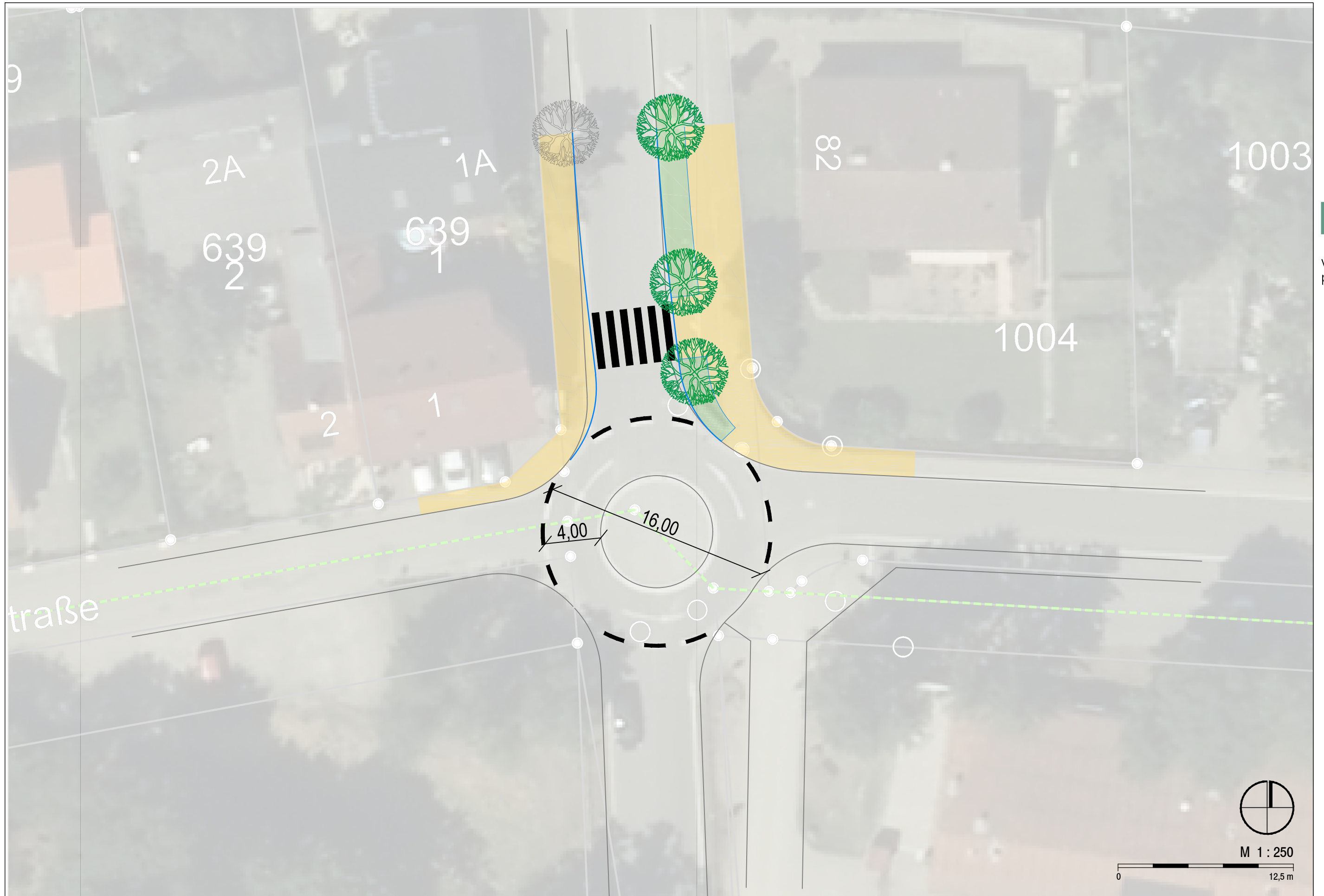
Entwurfstechnische Machbarkeit Minikreisverkehr Waldstraße/ In der Wolfshecke Variante 1
