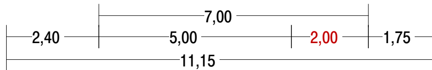
Variante Q6A Parken auf Fahrbahn (wechselseitig)
