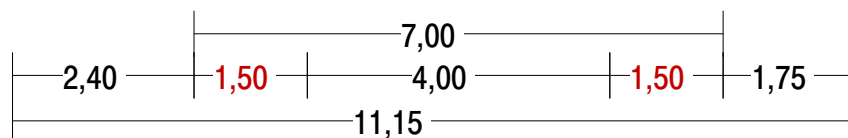
Variante Q6B beidseitiger Schutzstreifen ohne Parken
