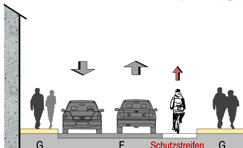
Variante Q1B Parken auf Fahrbahn (wechselseitig mit Ausweichstellen)
