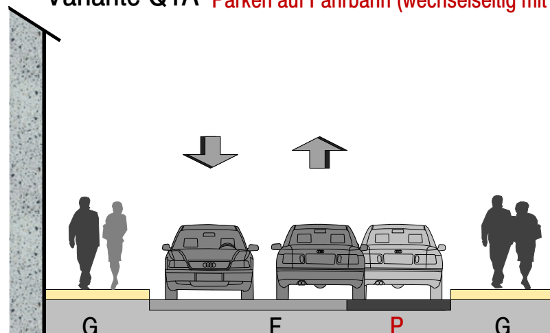
Variante Q1A Parken auf Fahrbahn (wechselseitig mit Ausweichstellen für Schwerverkehr)
